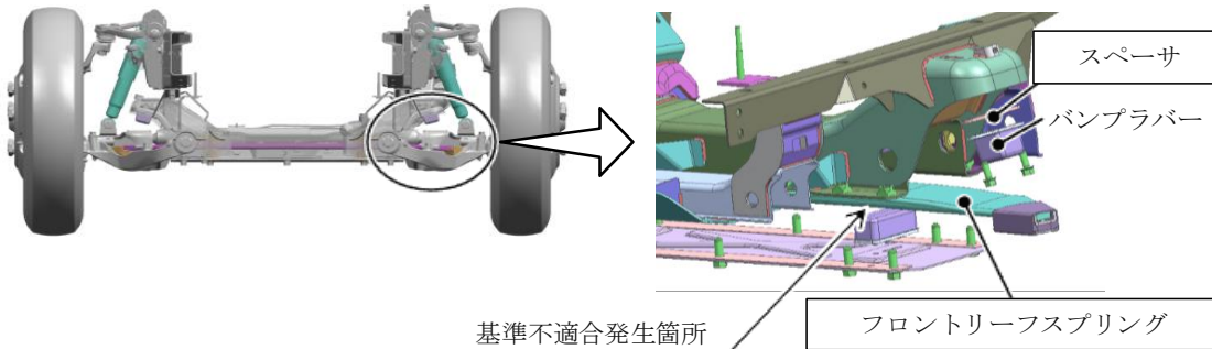
前輪緩衝装置全体図
